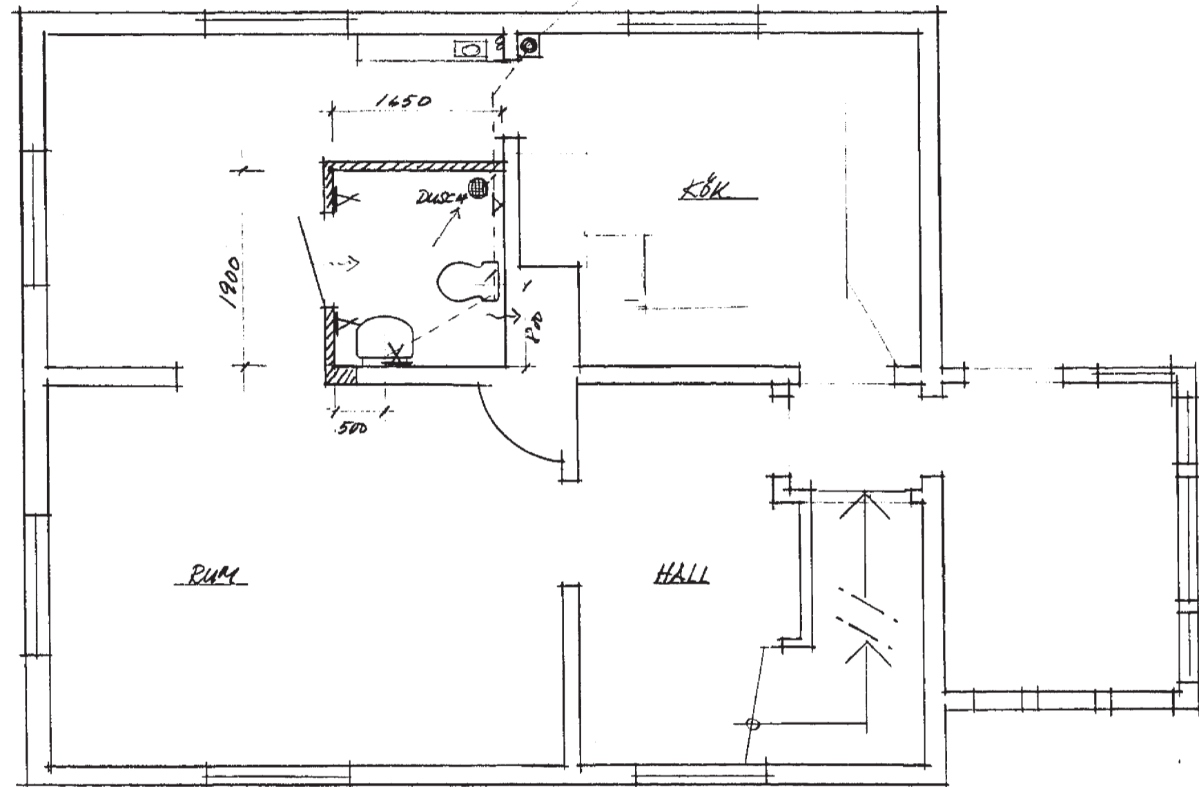
PLAN TOTTENVÅNING
