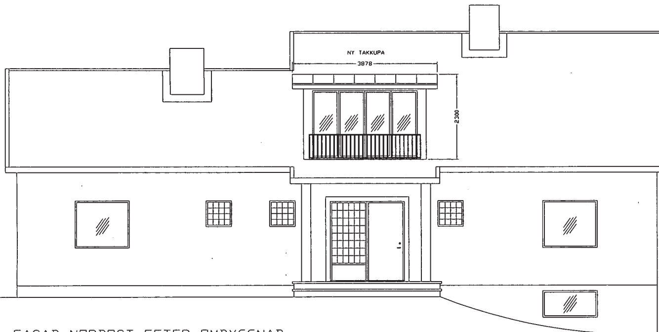
FASAD NÖRDBÖST EFTER ÖMÖBYGGNAD
